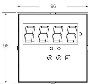
Voltmeter VM1-10
